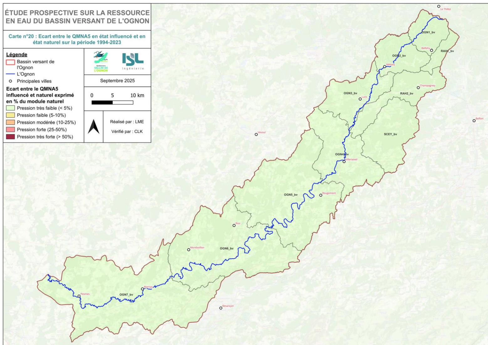
Figure 58: Ecart entre le QMNA5 naturel et influencé sur la période 1994-2023
