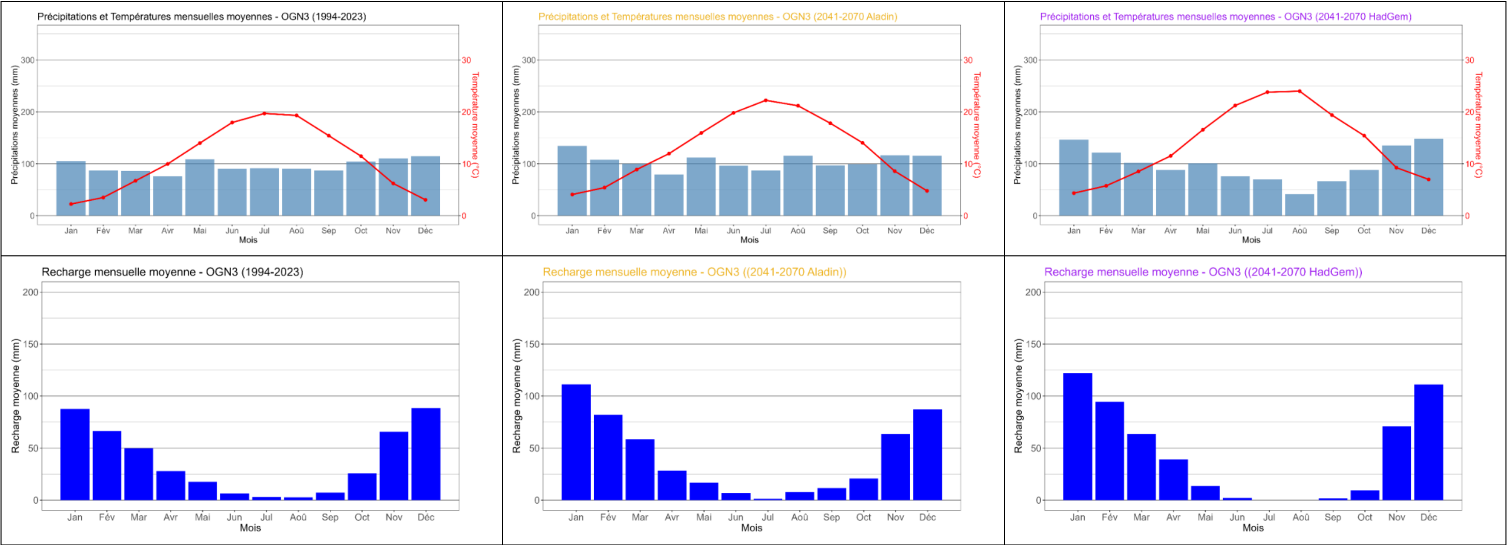
Figure 60: Evolution des précipitations, températures et recharge sur une année-type selon la période et le modèle pour OGN3
