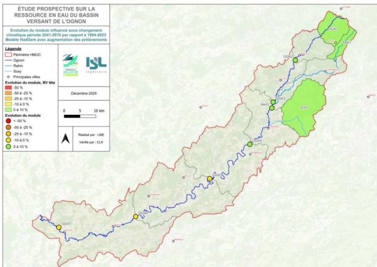
Figure 52: Evolution du module influencé en état futur (modèle HadGem augmentation) par rapport à l'état actuel
