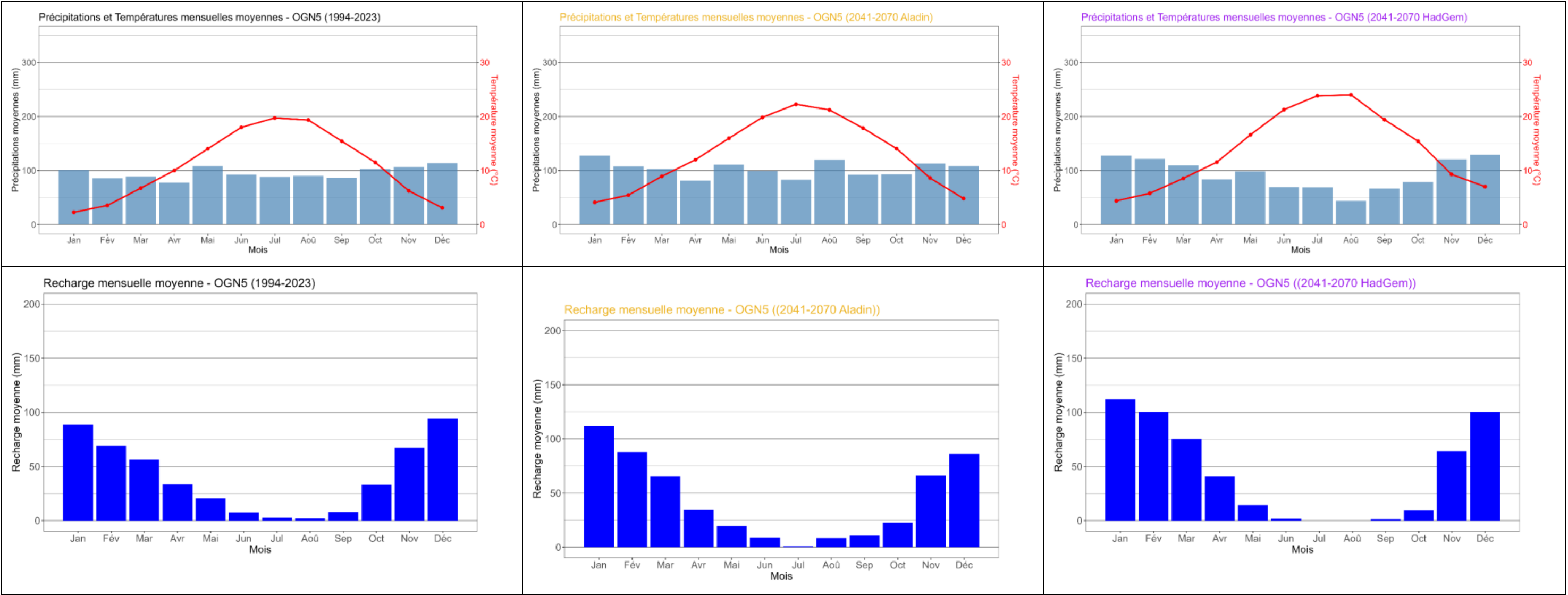
Figure 64: Evolution des précipitations, températures et recharge sur une année-type selon la période et le modèle pour OGN5
