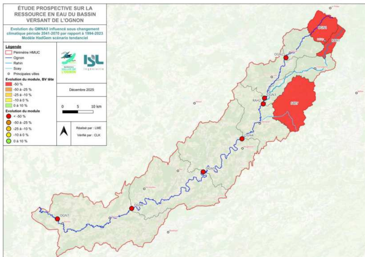
Figure 54: Evolution du QMNA5 influencé en état futur (modèle HadGem tendanciel) par rapport à l'état actuel
