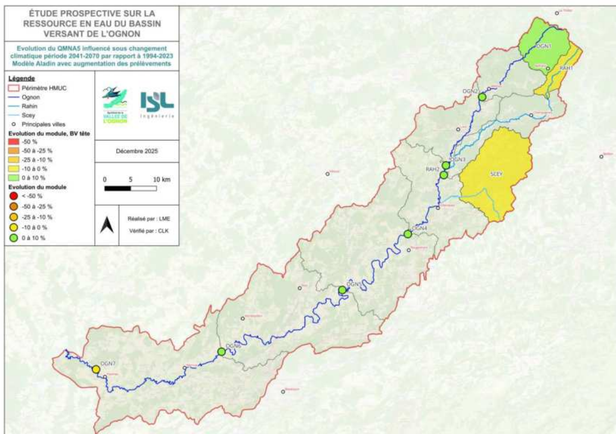
Figure 48 : Evolution du QMNA5 influencé en état futur (modèle Aladin augmentation) par rapport à l'état actuel
