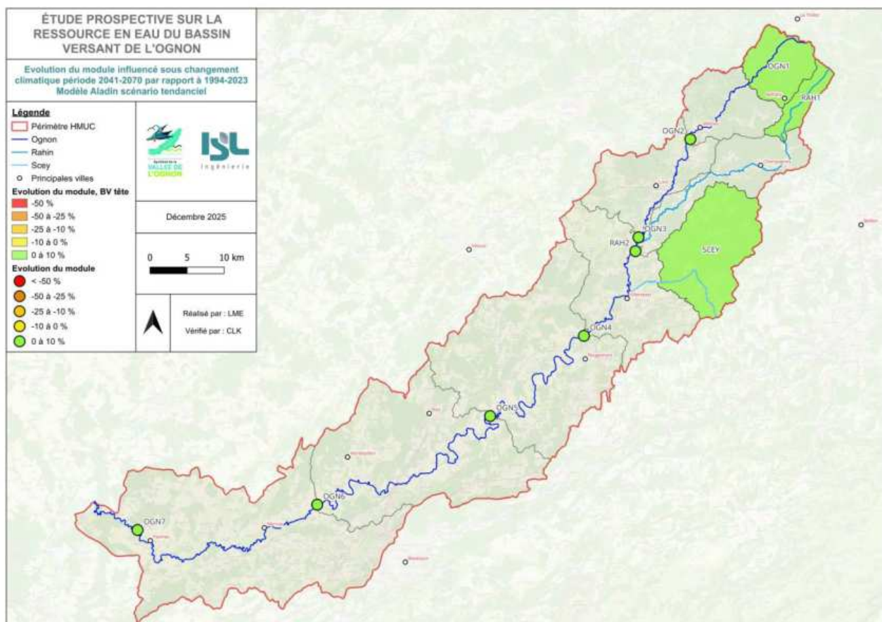
Figure 44: Evolution du module influencé en état futur (modèle Aladin tendanciel) par rapport à état actuel
