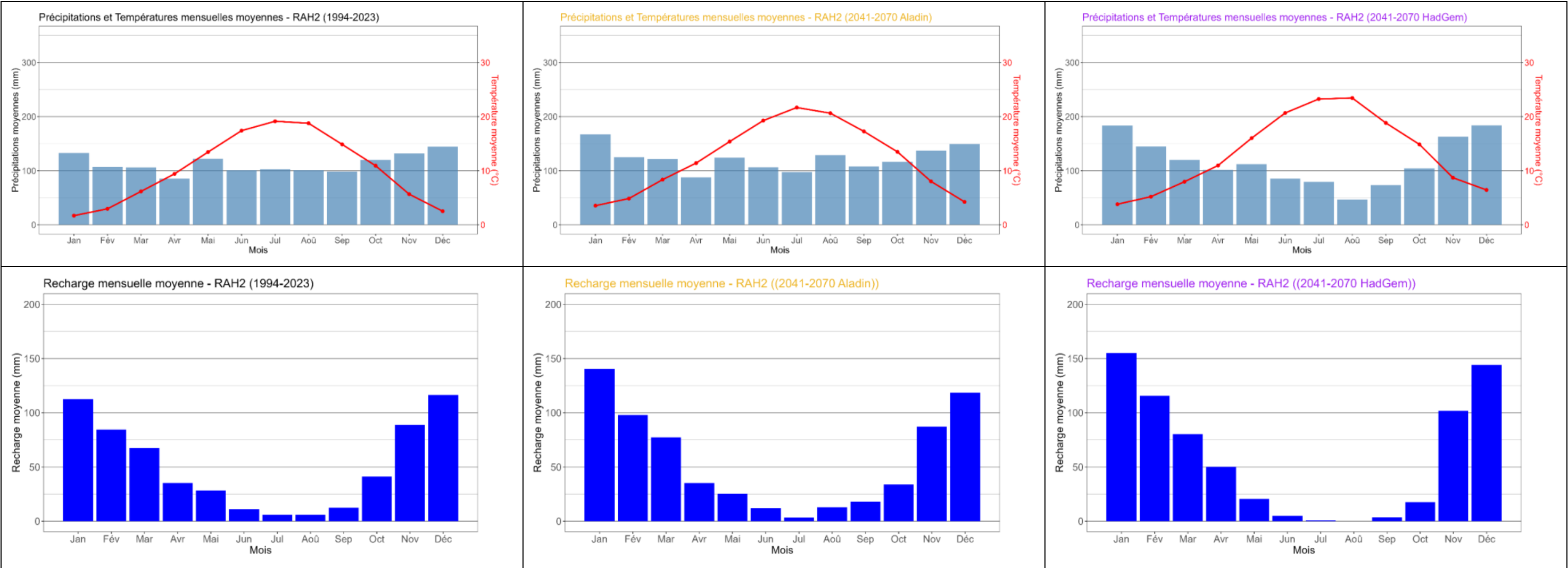
Figure 70: Evolution des précipitations, températures et recharge sur une année-type selon la période et le modèle pour RAH2
