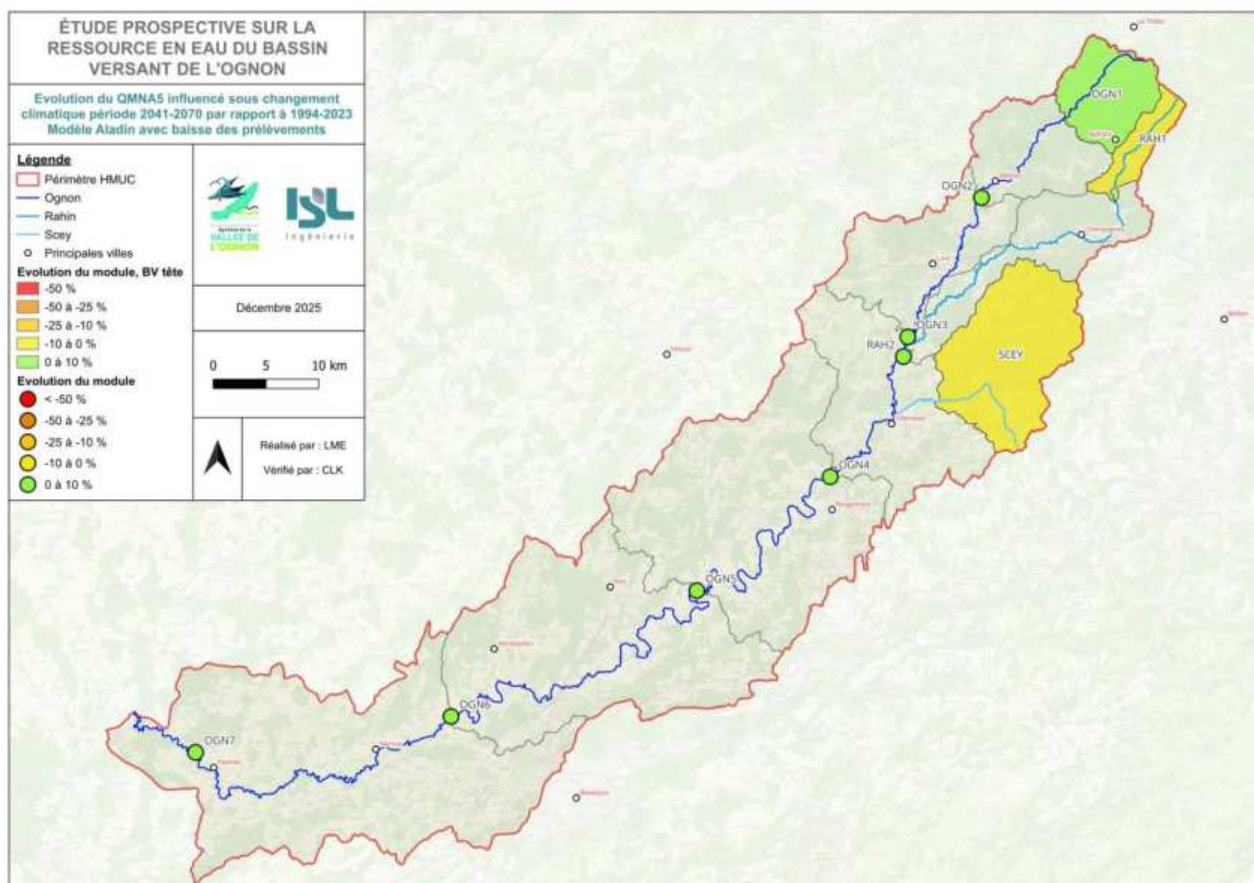
Figure 49 : Evolution du QMNA5 influencé en état futur (modèle Aladin baisse) par rapport à l'état actuel
