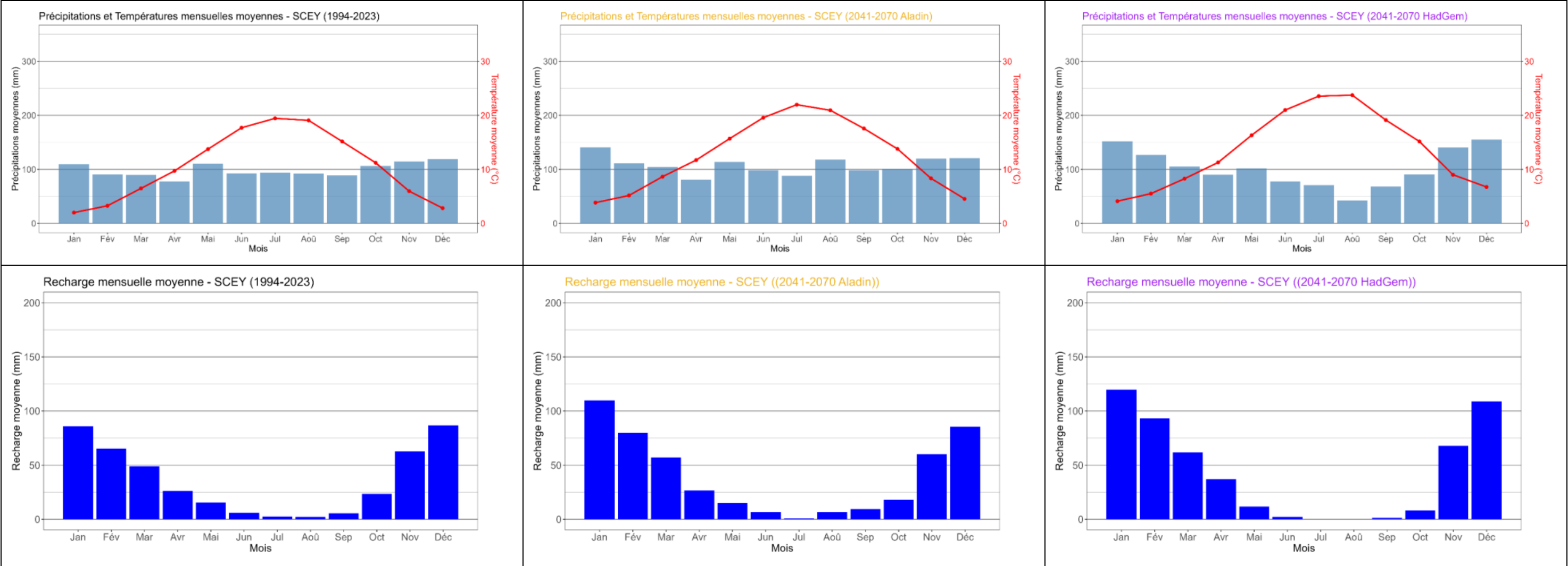
Figure 72: Evolution des précipitations, températures et recharge sur une année-type selon la période et le modèle pour SCEY
