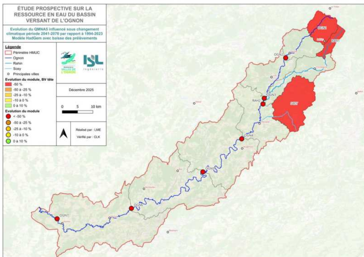
Figure 56: Evolution du QMNA5 influencé en état futur (modèle HadGem baisse) par rapport à l'état actuel
