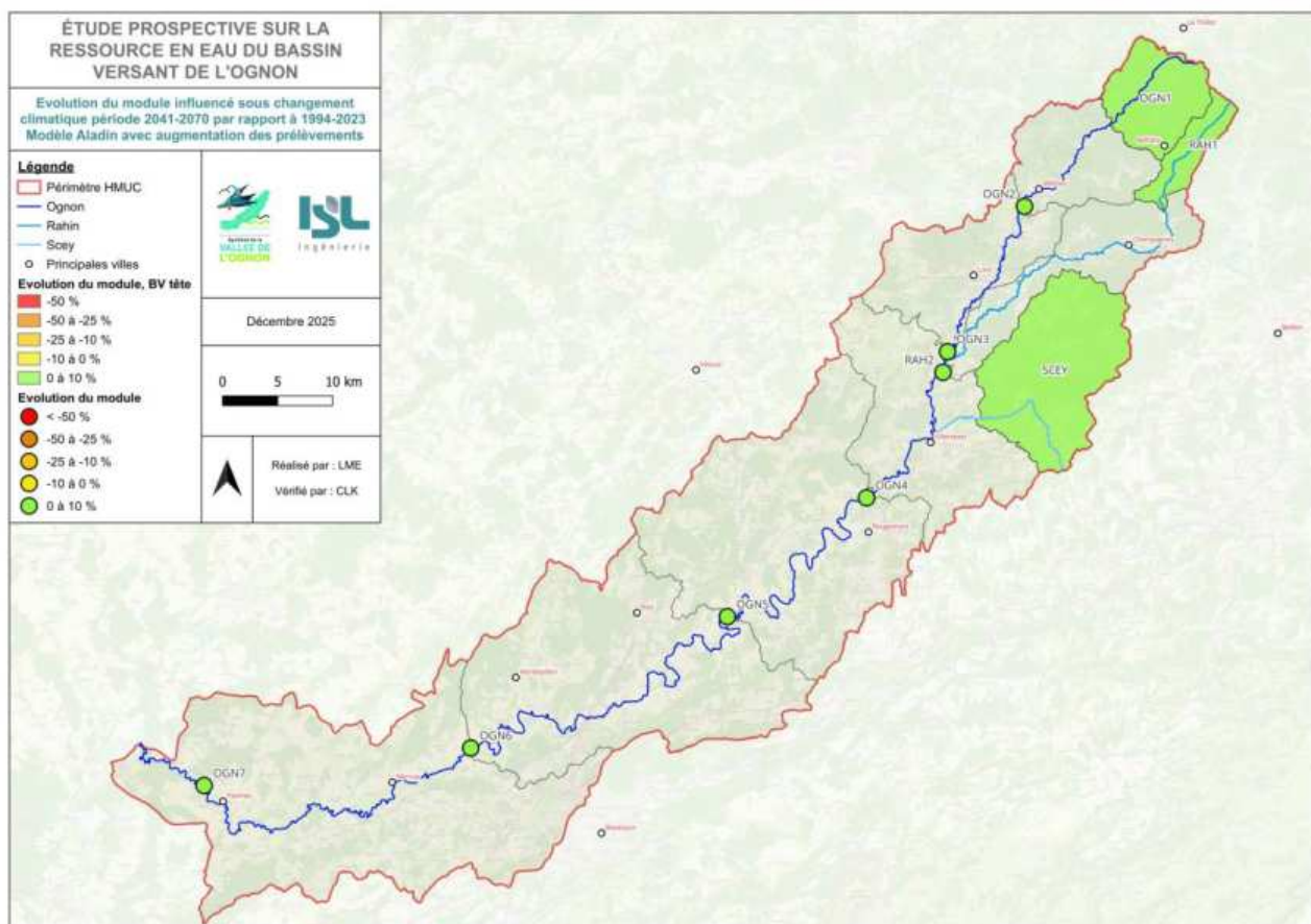
Figure 45: Evolution du module influencé en état futur (modèle Aladin augmentation) par rapport à l'état actuel
