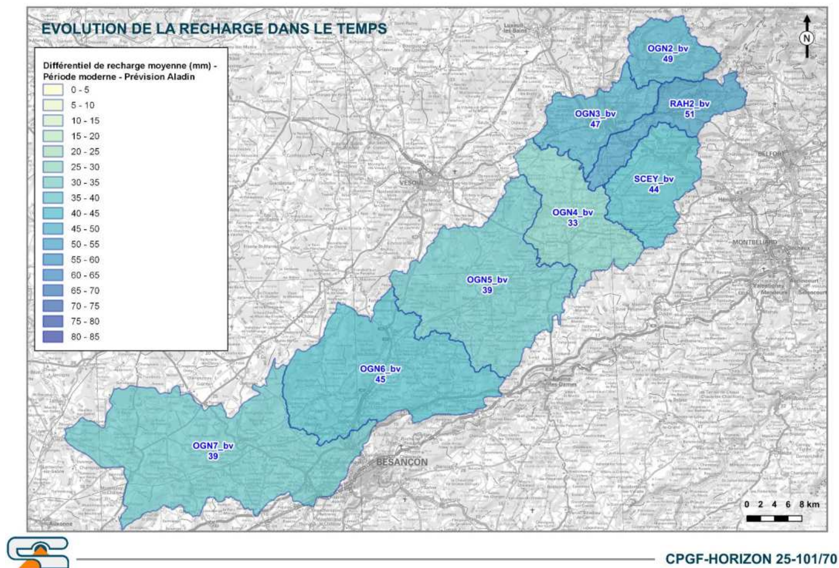
Figure 31: Evolution de la recharge basée sur modèle Aladin par rapport à la période moderne 1994-2023
