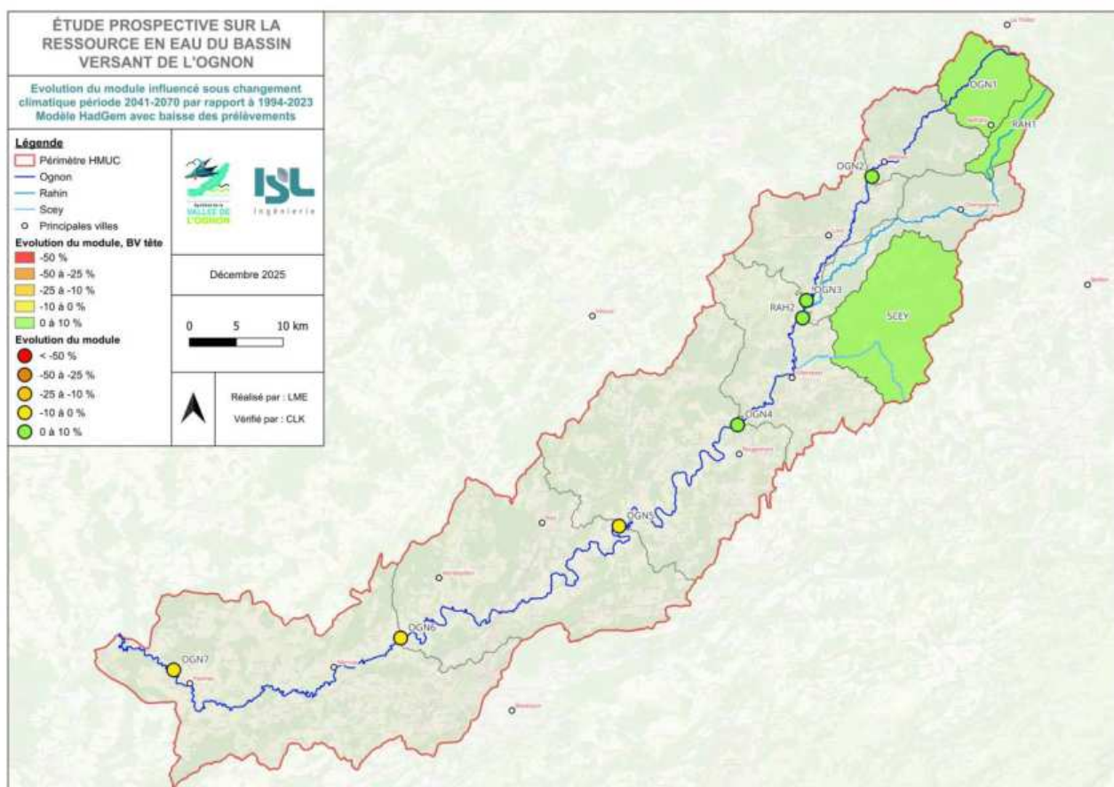
Figure 53: Evolution du module influencé en état futur (modèle HadGem baisse) par rapport à l'état actuel
