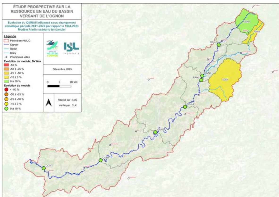
Figure 47: Evolution du QMNA5 influencé en état futur (modèle Aladin tendanciel) par rapport à l'état actuel
