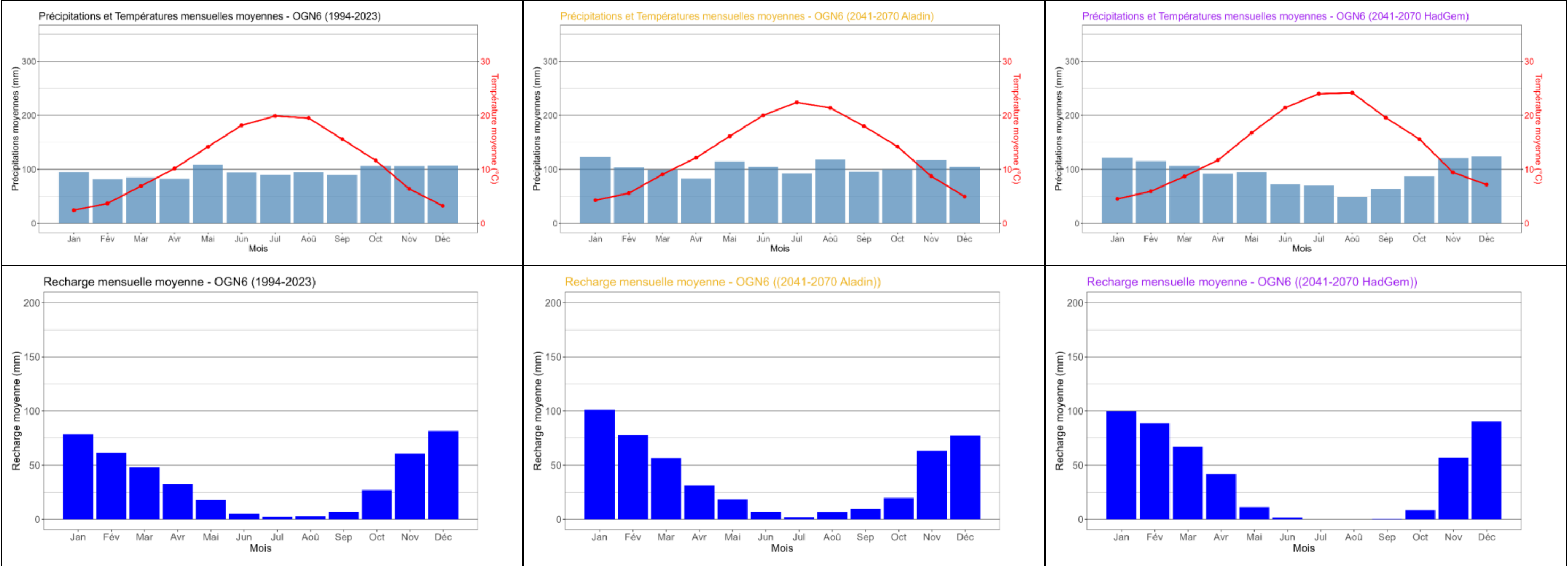
Figure 66: Evolution des précipitations, températures et recharge sur une année-type selon la période et le modèle pour OGN6
