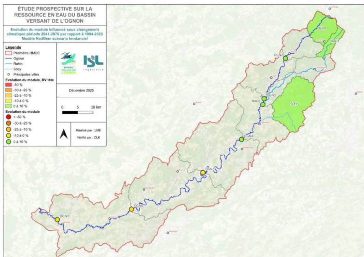
Figure 51: Evolution du module influencé en état futur (modèle HadGem tendanciel) par rapport à l'état actuel
