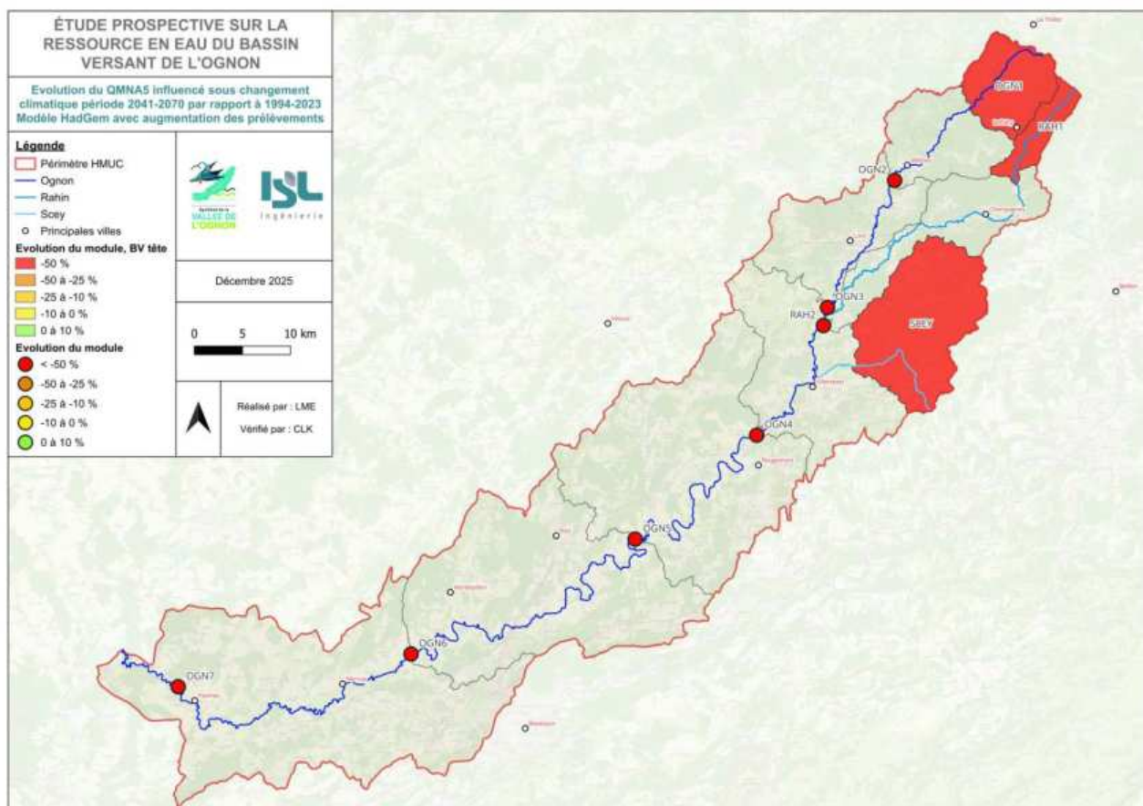
Figure 55: Evolution du QMNA5 influencé en état futur (modèle HadGem augmentation) par rapport à l'état actuel
