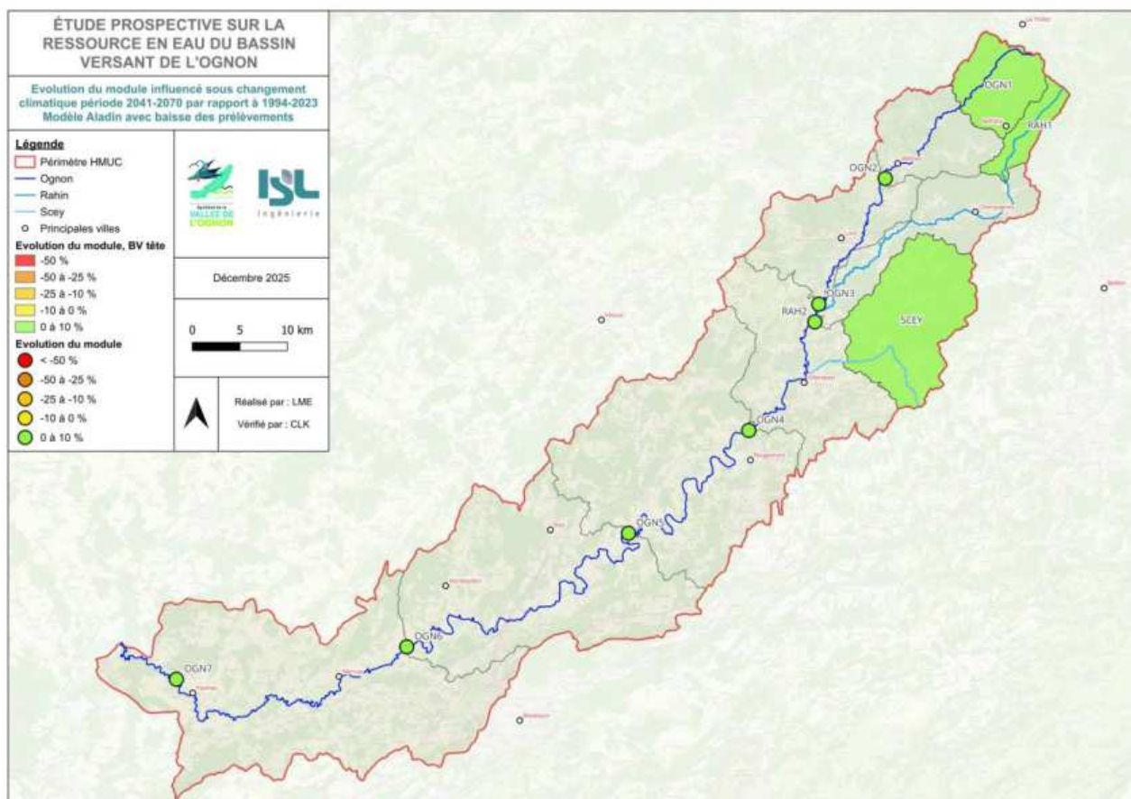
Figure 46: Evolution du module influencé en état futur (modèle Aladin baisse) par rapport à l'état actuel
