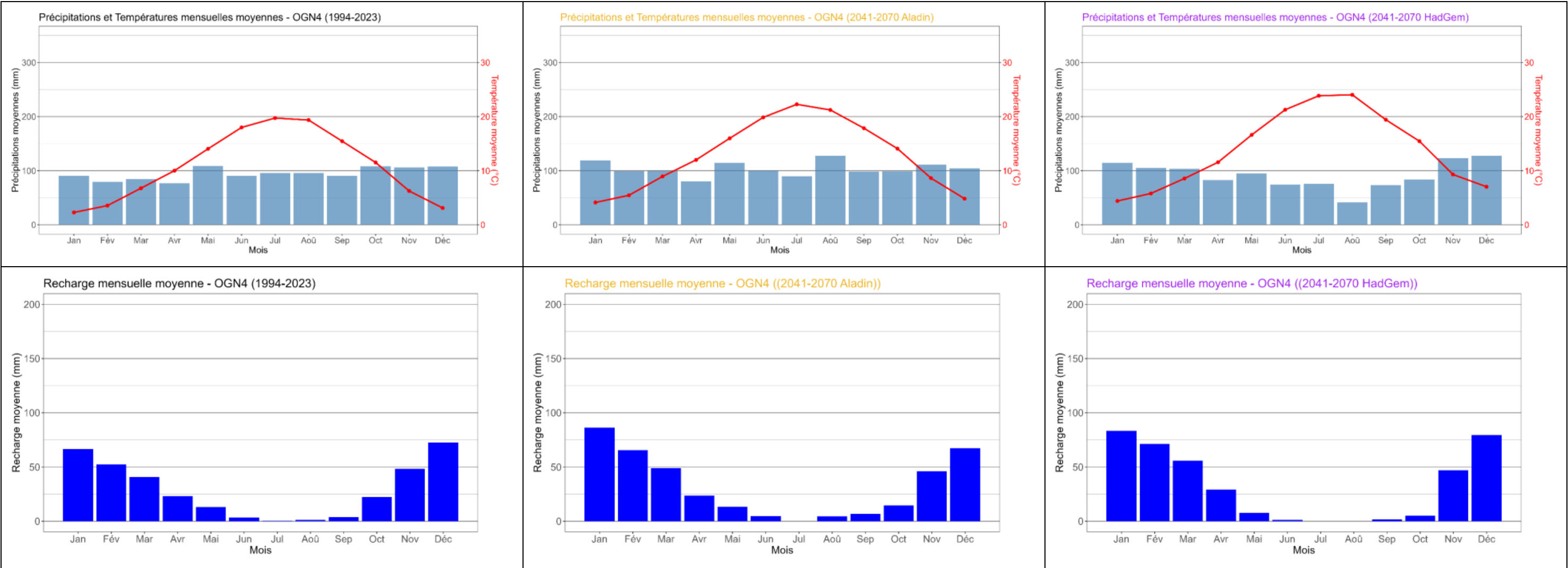
Figure 62: Evolution des précipitations, températures et recharge sur une année-type selon la période et le modèle pour OGN4
