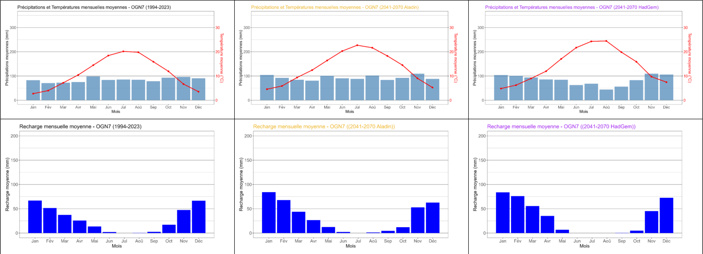
Figure 68: Evolution des précipitations, températures et recharge sur une année-type selon la période et le modèle pour OGN7
