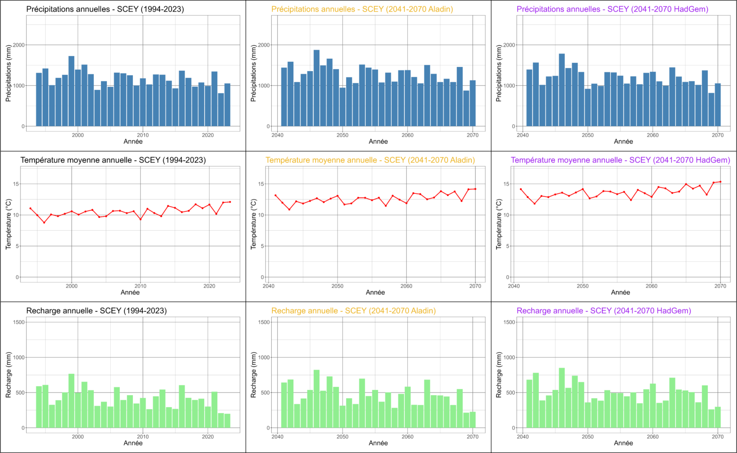
Figure 71: Evolution des précipitations, températures et recharge au pas de temps annuel selon la période et le modèle pour SCEY
